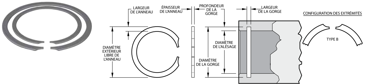
Dimensions des produits Toutes les dimensions sont exprimées en pouces sauf spécification contraire.
