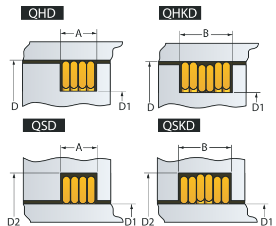
Dimensions des produits Toutes les dimensions sont exprimées en millimètres sauf spécification contraire.
