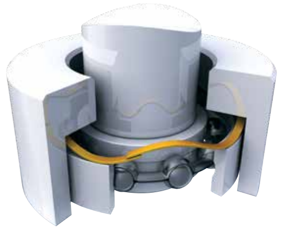
G. ベアリング プリロード
