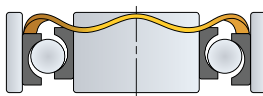
プリロードを持つベ어링:ボール コンプリメントとベ어링 レースが確実に合致し、振動と磨耗を低減または除去。
